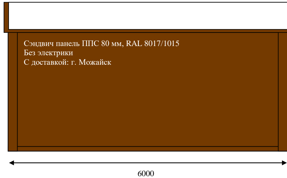
Вид сзади
